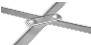
Plat/Plat kruisverbinding
